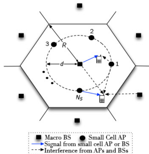
그림 1. 이종 이동통신 네트워크 Fig. 1 Heterogeneous Mobile Communication Network
