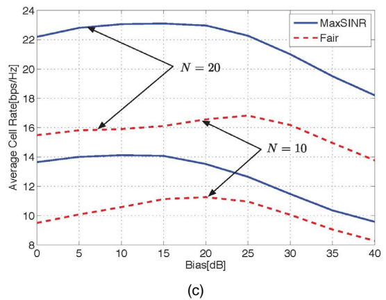
그림 2. 셀 확장 편향치에 따른 평균 셀 전송 효율 (a) N_s = 5 (b) N_s = 10 (c) N_s = 20 Fig. 2 Average Cell Rate For CREB Values (a) N_s = 5 (b) N_s = 10 (c) N_s = 20
